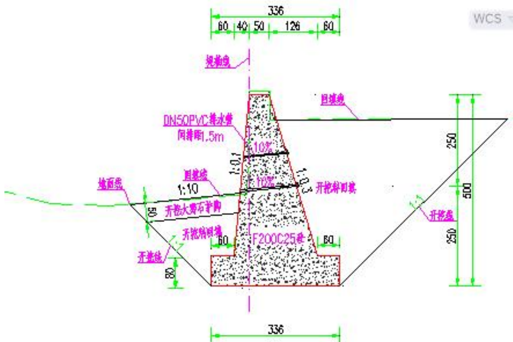
方案 3: F200C25 砼仰斜式堤防
