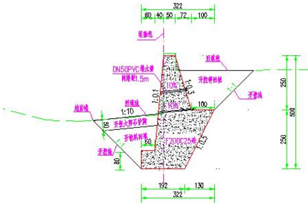
方案 2: F200C25 砼重力式堤防
